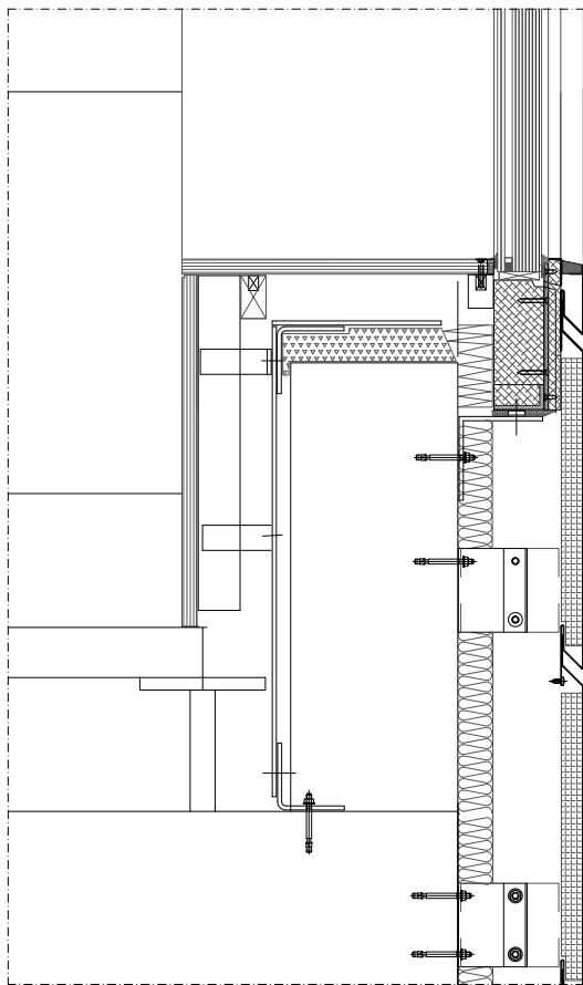
DETTAGLIO B
