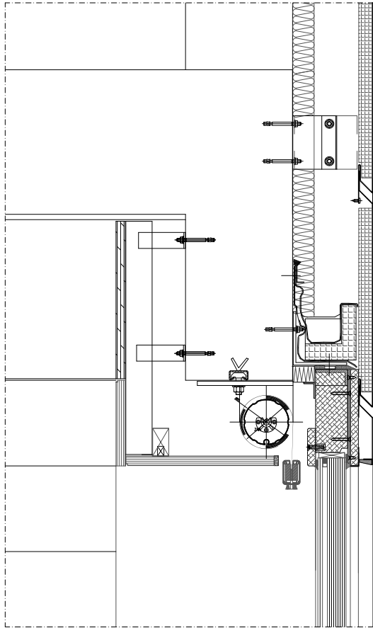
DETTAGLIO C
